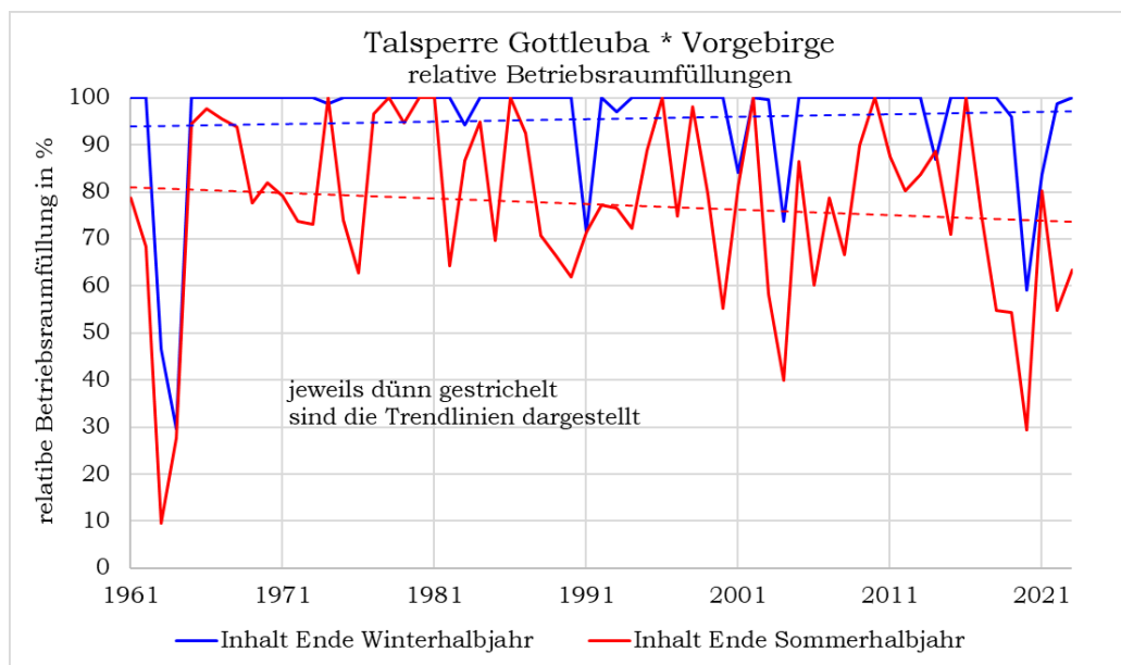
Abbildung 1: Relative Betriebsraumfüllstände der Talsperre Gottleuba im Naturraum sächsisches Vorgebirge von 1961 – 2023
