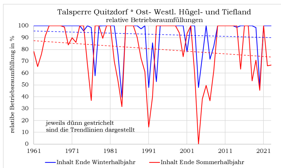
Abbildung 3: Relative Betriebsraumfüllstände der Talsperre Quitzdorf im Naturraum Ost- Westl. Hügel- und Tiefland, von 1961 – 2023
