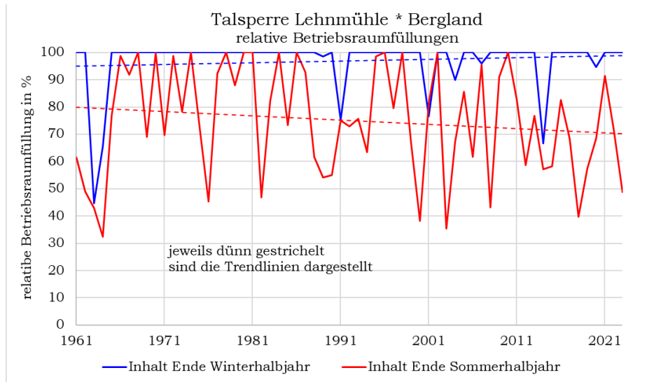
Abbildung 5: Relative Betriebsraumfüllstände der Talsperre Lehmühle im Naturraum sächsisches Bergland, von 1961 – 2023
