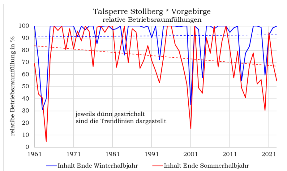
Abbildung 4: Relative Betriebsraumfüllstände der Talsperre Stollberg im Naturraum sächsisches Vorgebirge, von 1961 – 2023
