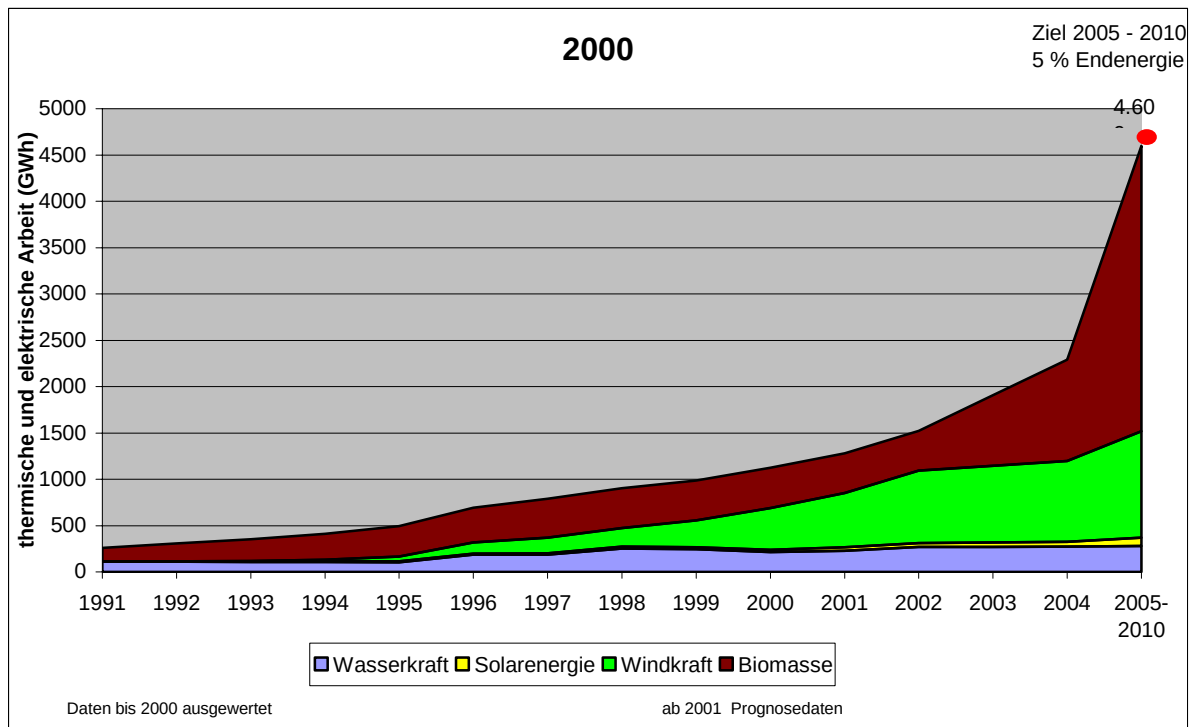
Abb. 15: Stand und Ziel der Nutzung erneuerbarer Energien in Sachsen – 2000 Quellen: Klimaschutzprogramm des Freistaates Sachsen; LfUG, EEZ
