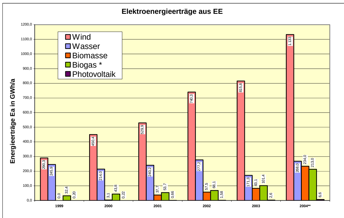
Abb. 14: Jahreselektroenergieerträge aus erneuerbaren Energien 1999 bis 2004
